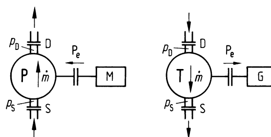
Bild 1-3 Fluidenergiemaschinen; symbolische Darstellung
