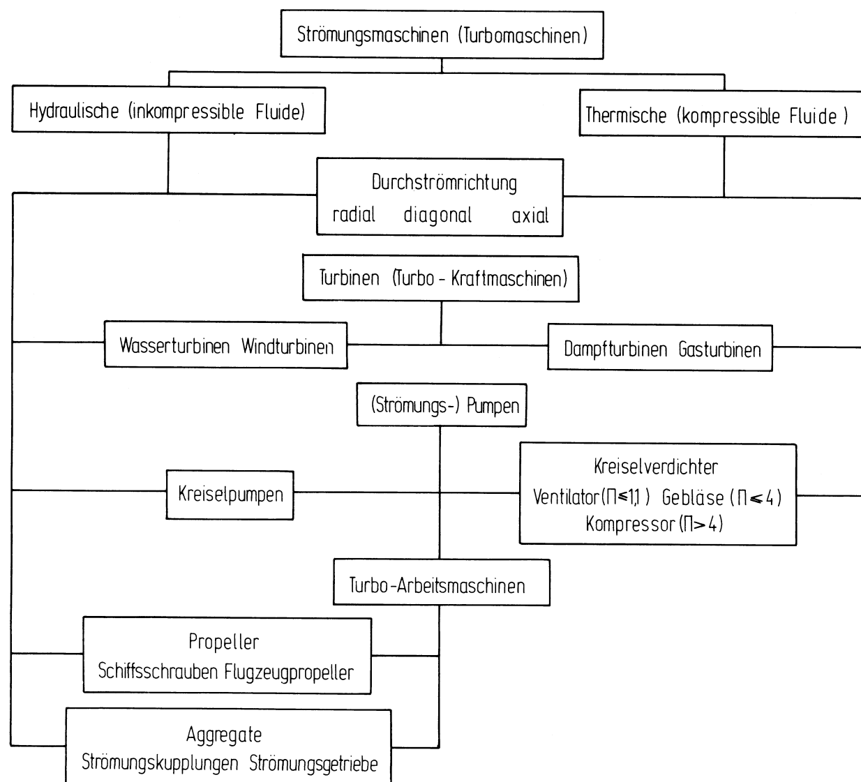
Bild 1-1 Aufteilung der Strömungsmaschinen (Turbomaschinen → Turbo 1) ... Kreisel) nach Anwendung (AM, KM), Arten (HyM, ThM), Bauformen (radial, diagonal, axial) und Typen (Druckverhältnis \Pi )
