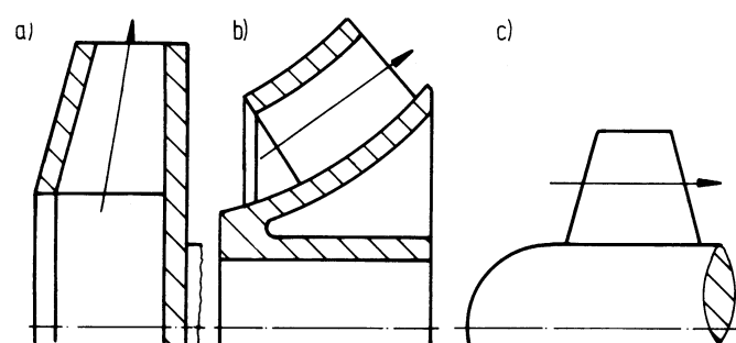
Bild 1-2 Laufradausführungen (Prinzip-Darstellungen) a) radial, b) diagonal (halbaxial), c) axial
